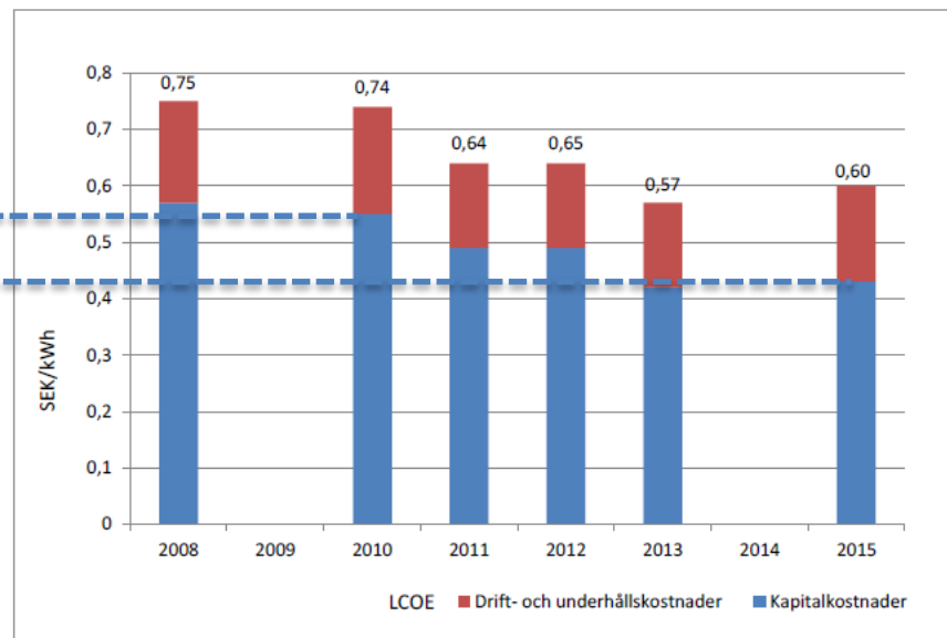
Figur 2.14 Utveckling av elproduktionskostnaderna i Sverige 2008-2015. Källa: Levelised Cost of Energy for Swedish wind farms – an empirical study, Ernst&Young, feb 2015. Anm: För åren 2009 och 2014 fanns det för få projekt för att kunna redovisa någon kostnadsnivå.
